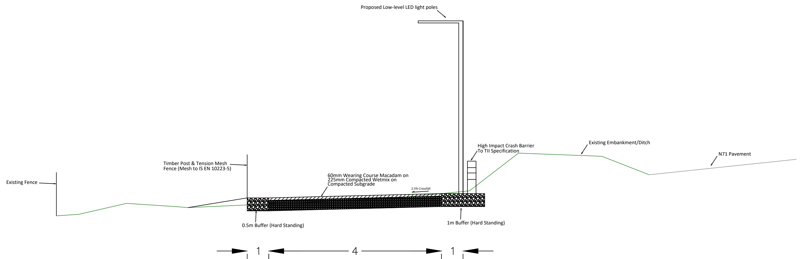
Section A-A
